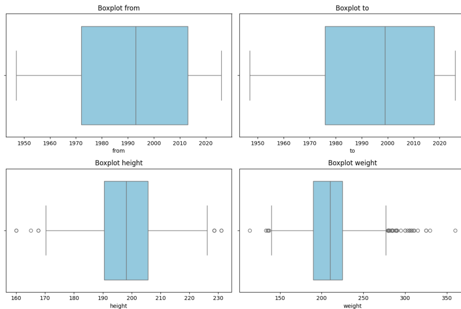
Gambar 1. Boxplot atribut numerik
