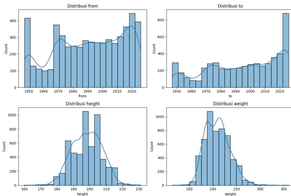
Gambar 2. Histogram atribut numerik
