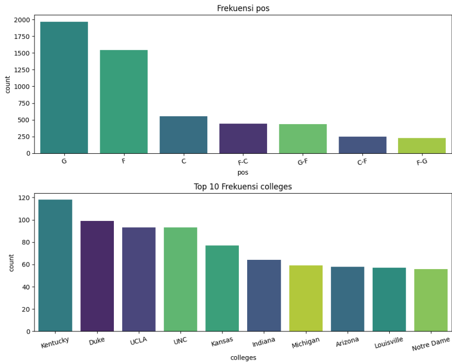
Gambar 3. Bar plot atribut kategorikal
